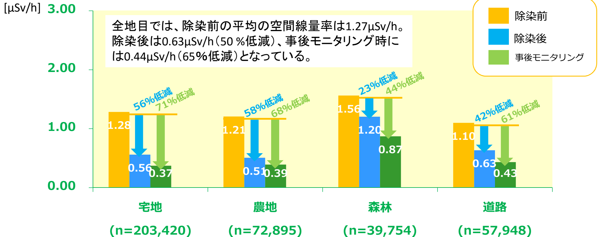
図. 宅地、農地、森林、道路の空間線量率の平均値(測定点データの集計)
