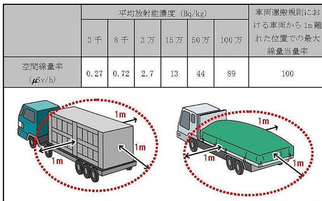
図 2.1.3-10 輸送車両から 1\text{m} の地点における空間線量率の試算例
