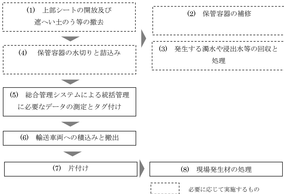
図 2.1.3-1 作業フロー
