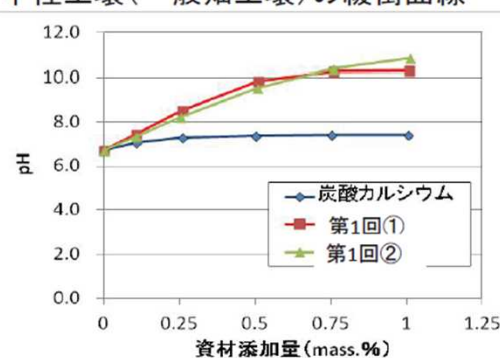
中性土壌(一般畑土壌)の緩衝曲線
