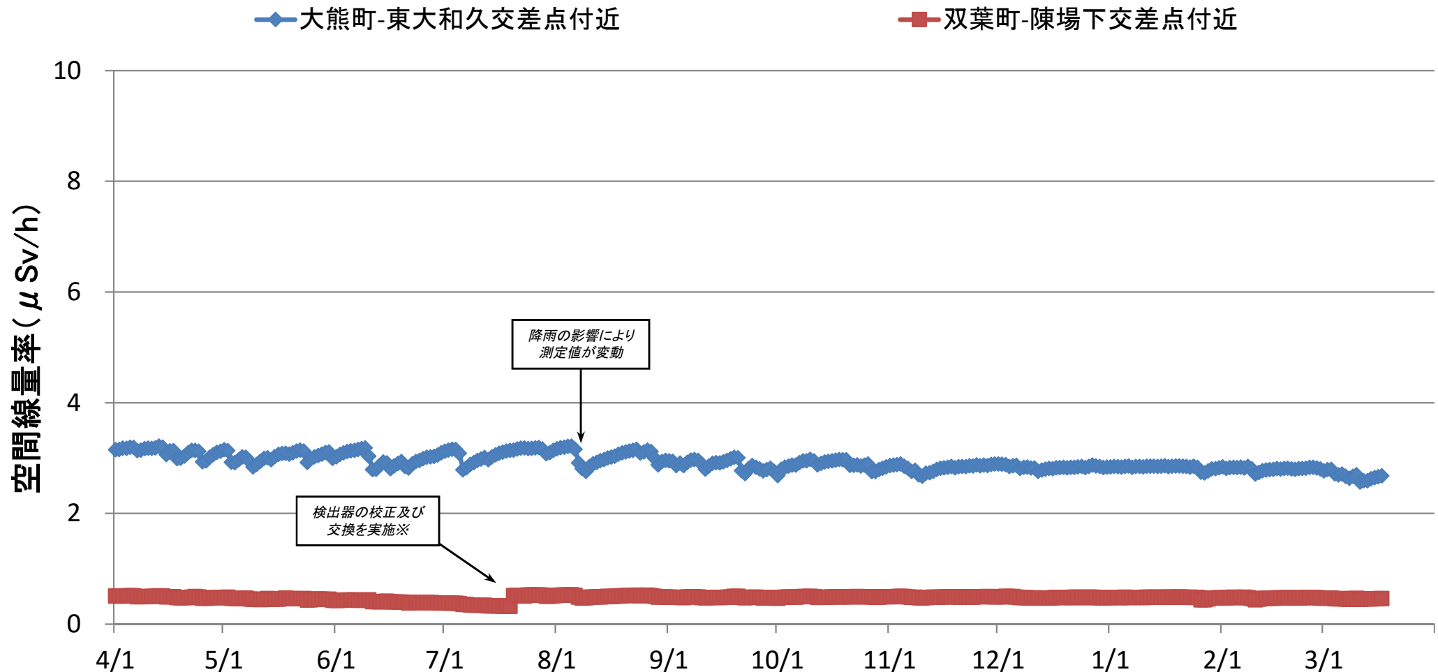
中間貯蔵施設区域境界における空間線量率の推移(連続測定) (2018年4月1日～2019年3月17日)
