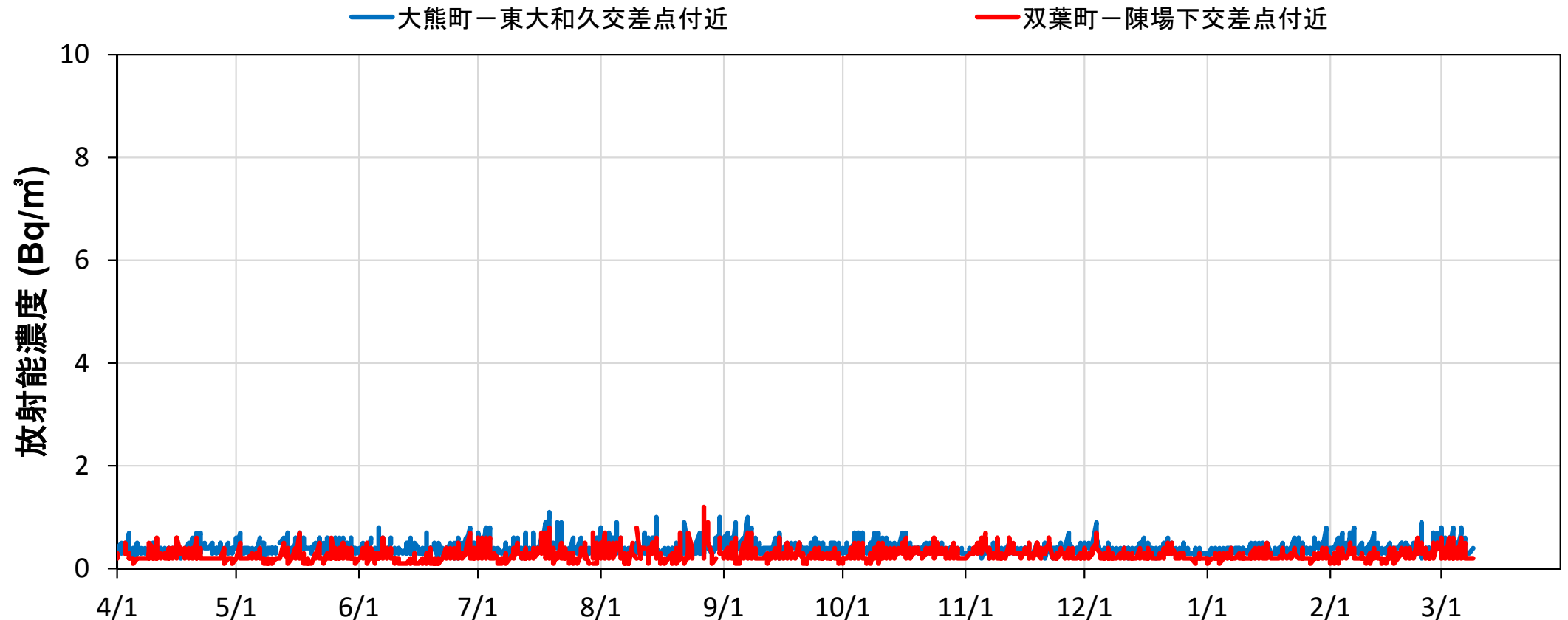
中間貯蔵施設区域境界における大気中の \beta 線の放射能濃度(連続測定) (2018年4月1日～2019年3月8日)
